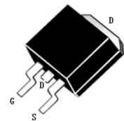
CS5N50A3/TO-263
